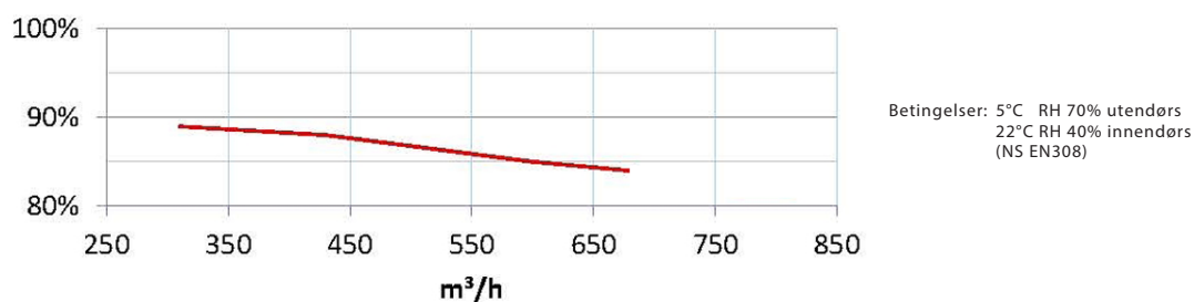
Temperaturvirkningsgrad AHU-550 BH/BV
