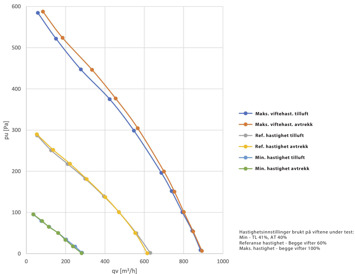
Diagram luftmengde/trykk
