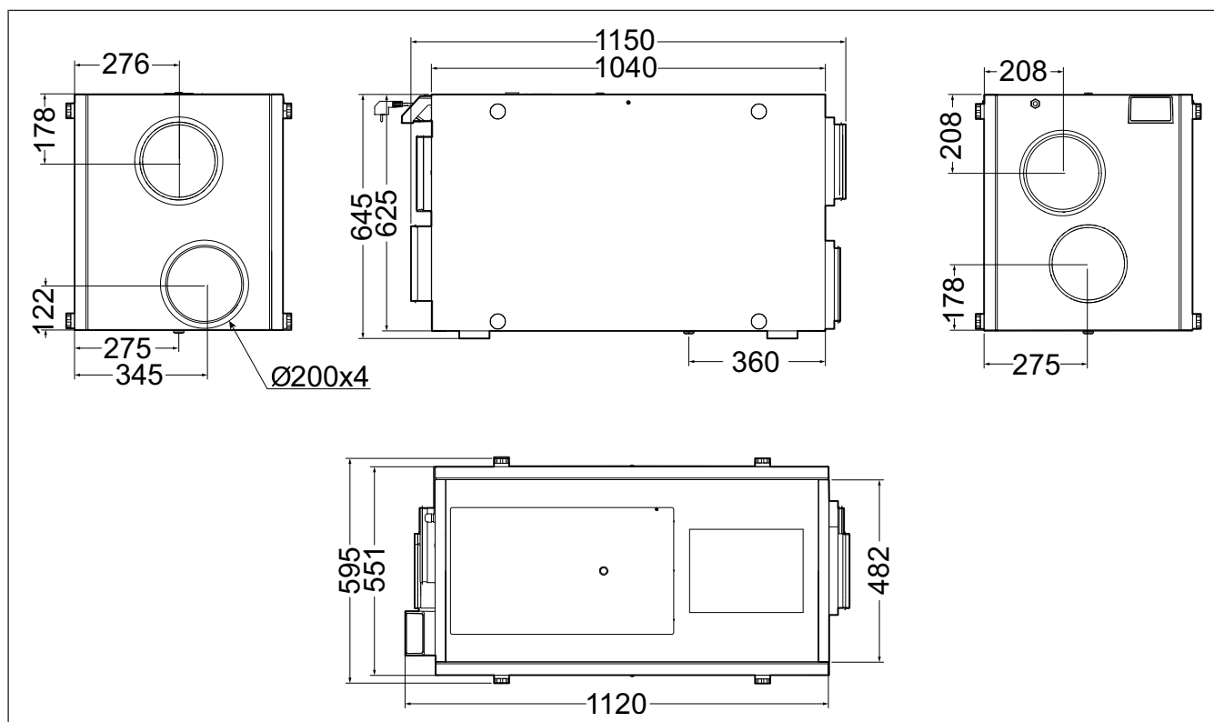
Fig. 2 SAVE VSR 500
