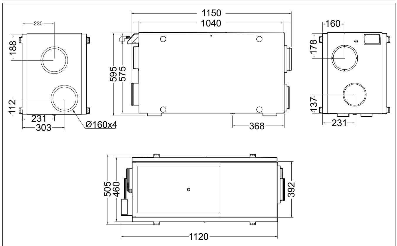
Fig. 1 SAVE VSR 300
